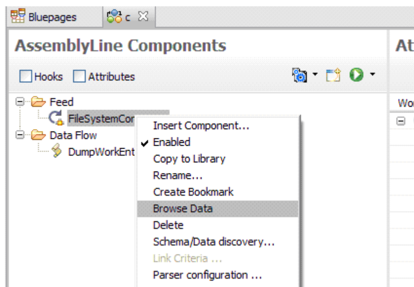
Figure 46. Data Browser
