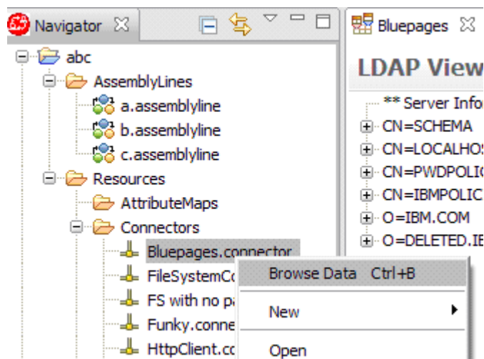
Figure 45. Data Browser
